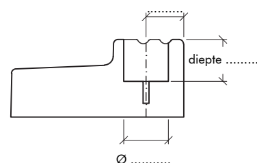
Boorgat niet door-en-door max. diepte 43mm
