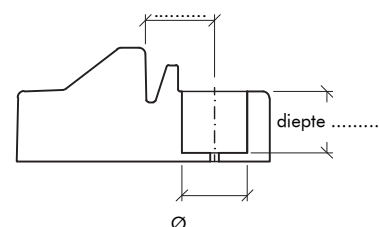
Boorgat niet door-en-door max. diepte 28mm
