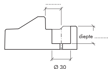
Boorgat niet door-en-door max. diepte 26mm
