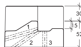
Boorgat niet door-en-door max. diepte 28mm
